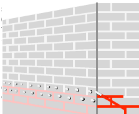
(injectiemethode t.b.v. Masterseal 1160 DPC)
